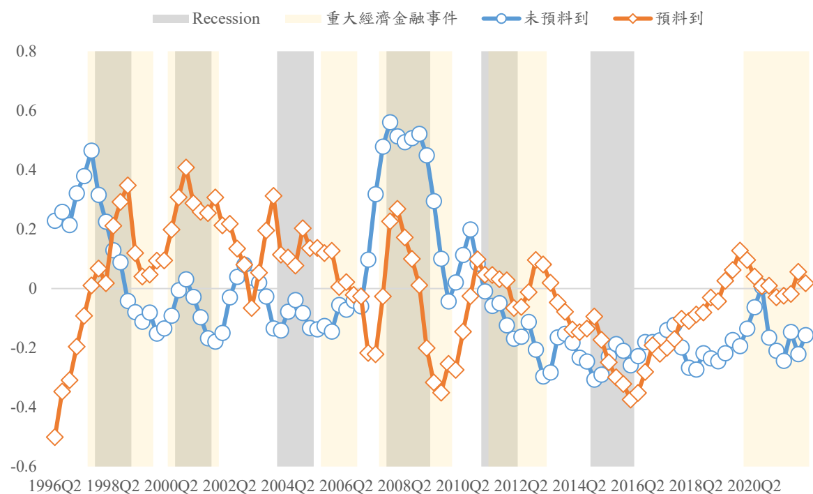
(B) 平滑化後(MA)數列
